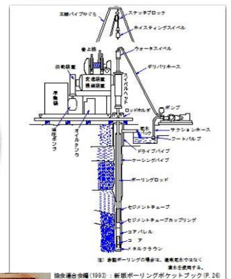
図 3.1.1 ボーリング機械概念図
